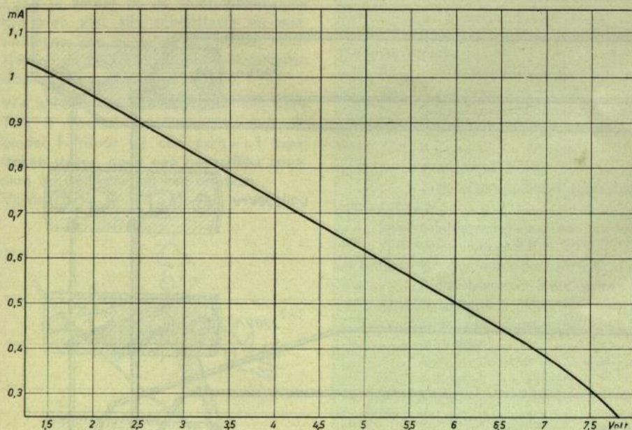
Stroom en spanning indien R1 = 8200 \Omega
