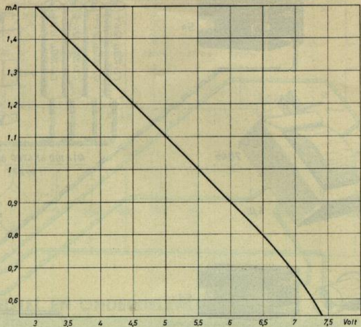
Stroom en spanning indien R1 = 4700 \Omega
